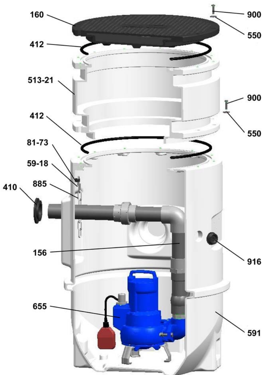
Vue éclatée installation transportable
